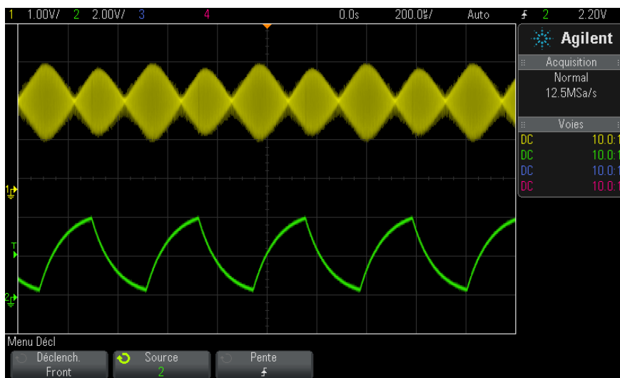
Figure 26 Modulation d'amplitude représentée à une intensité de 40%
