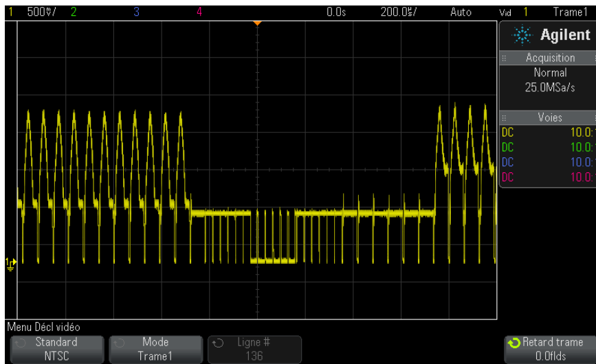
Figure 29 Déclenchement sur la trame 1
