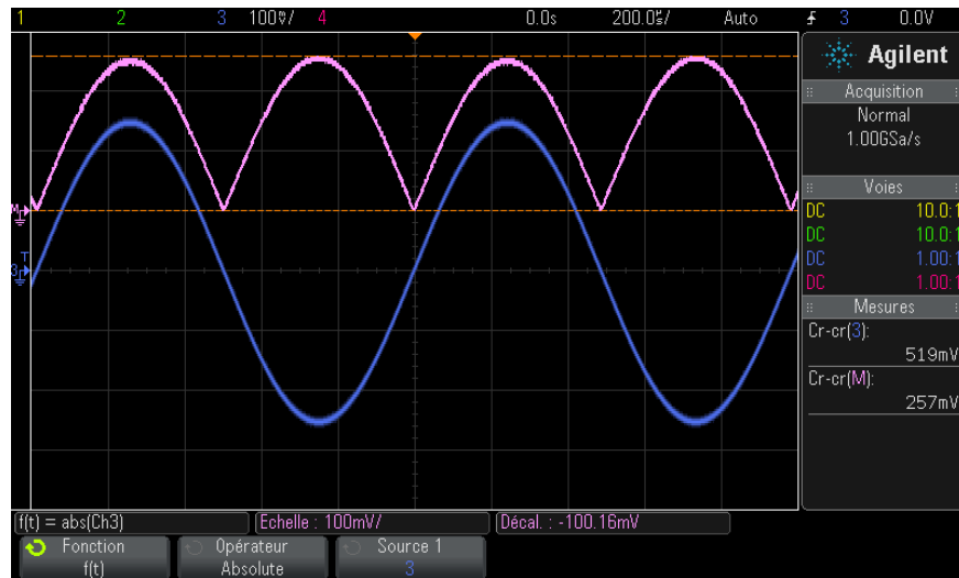
Figure 12 Exemple de valeur absolue
