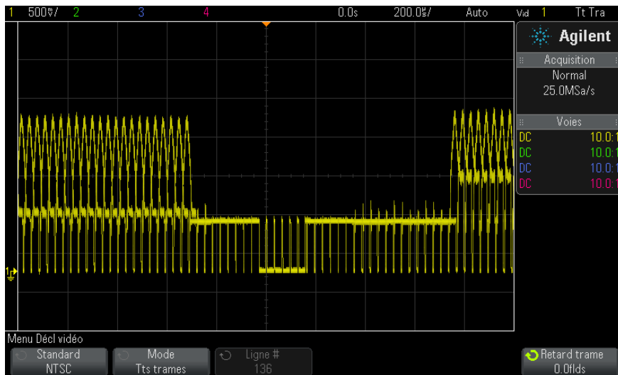
Figure 30 Déclenchement sur toutes les trames
