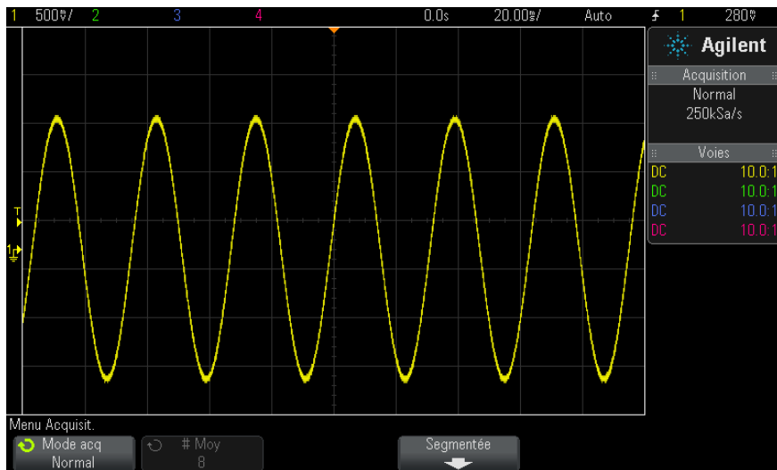
Figure 36 Sinusoïde avec impulsion transitoire, mode Normal
