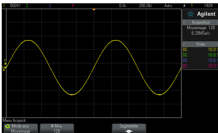
Figure 39 128 moyennes utilisées pour réduire le bruit aléatoire
