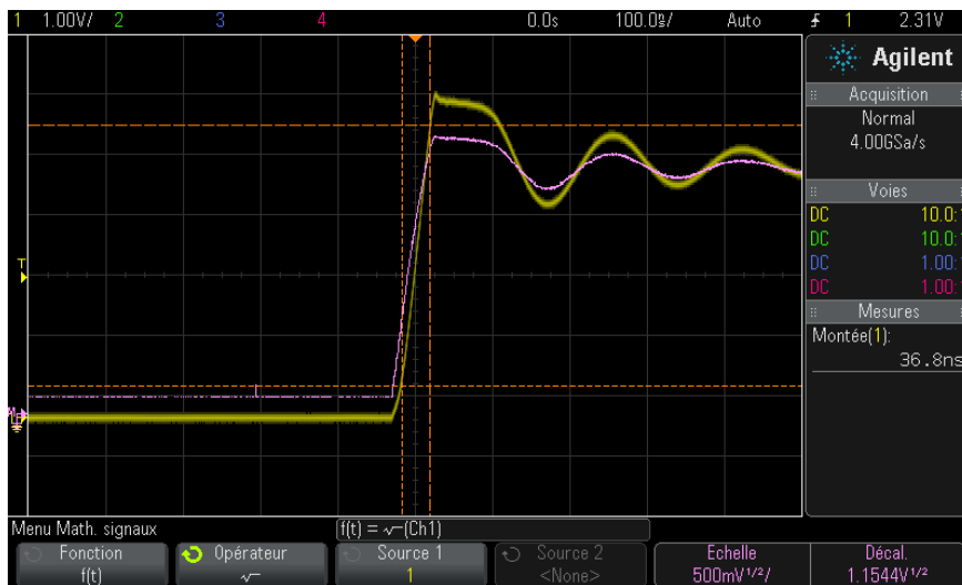
Figure 10 Exemple de fonction \sqrt{\quad} (Racine carrée)
